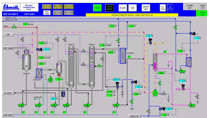
Wizualizacja procesu działania instalacji do usuwania alkoholu SIGMASKID
